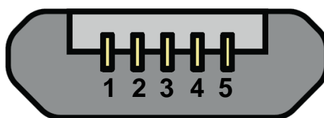
Рис. 2.5 Разъем micro-USB
