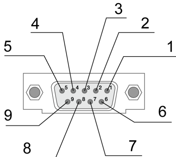
Рис. 2.5.1. Интерфейсный разъем
