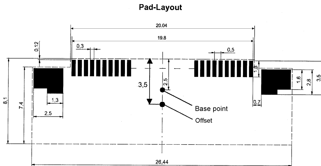
Figure 30: PCB ZIF connector
