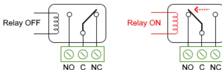
Рис. 4. Релейные выходы контроллера Socket-3.
