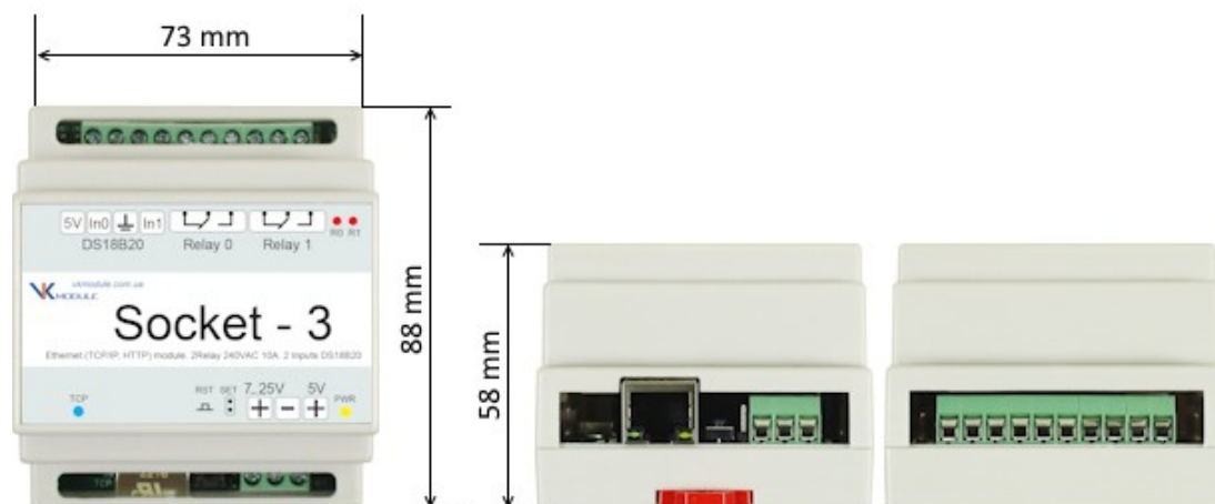
Рис.1. Внешний вид контроллера Socket-3.
