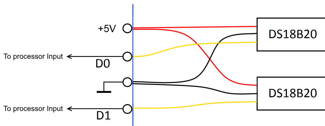
Рис. 3. Подключение датчиков температуры.
