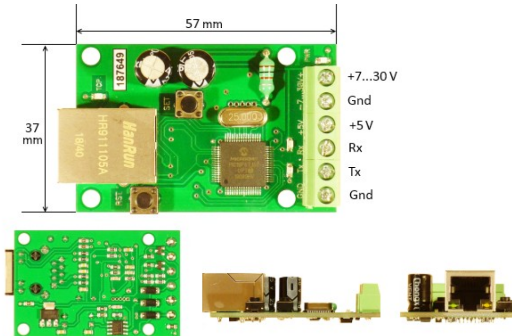
Рис.1. Зовнішній вигляд перетворювача VTR-E/TTL.
