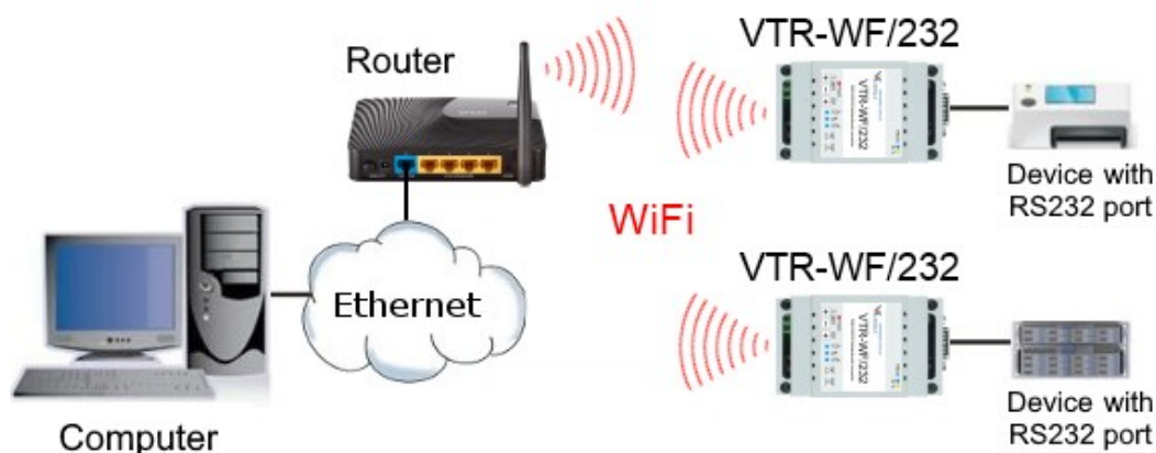
Рис 1. Підключення VTR-WF/232 до комп'ютера.
