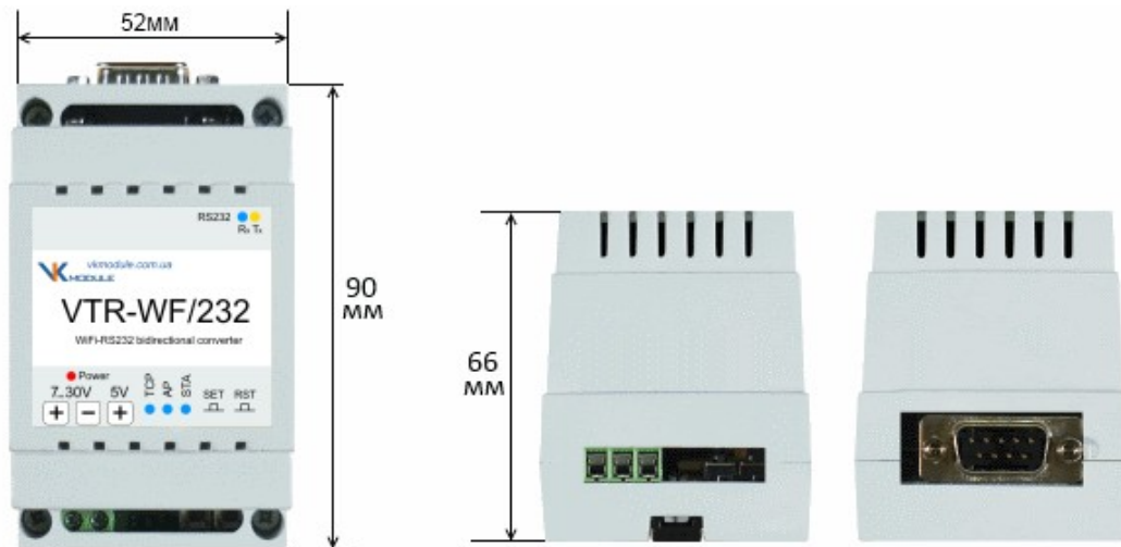
Рис. 4. Зовнішній вигляд перетворювача VTR-WF/232.
